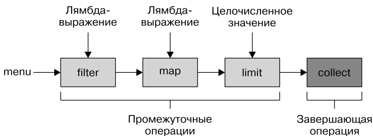
Рис. 4.5. Промежуточные и завершающие операции
