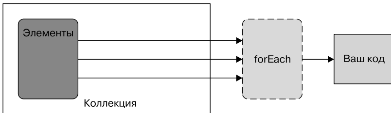
Рис. 4.4. Внешняя и внутренняя итерация
