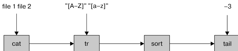
Рис. 1.2. Обработка потока данных командами Unix
