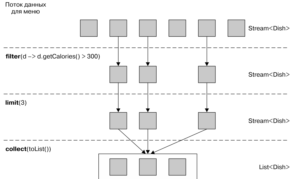
Рис. 5.3. Усечение потока данных
