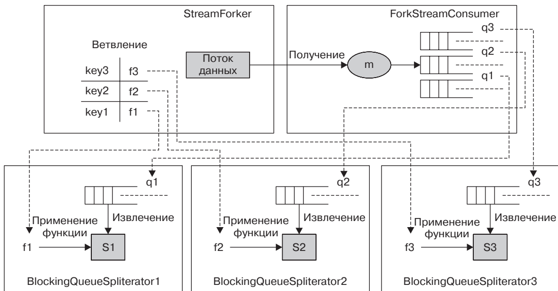
Рис. В.2. Составные части класса StreamForker
