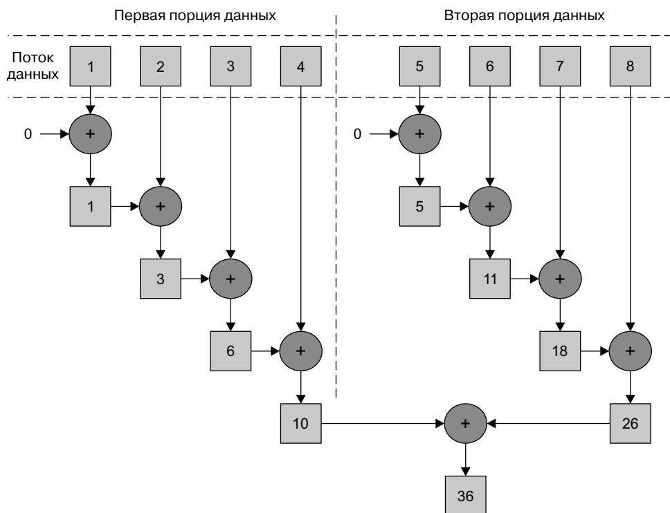
Рис. 7.1. Параллельная операция свертки
