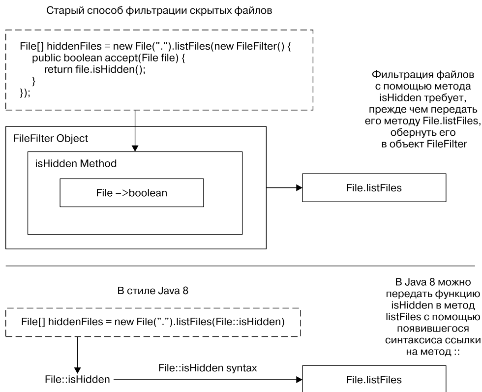
Рис. 1.4. Передача ссылки на метод File::isHidden в метод listFiles
