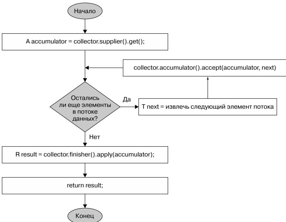
Рис. 6.7. Логические шаги процесса последовательной свертки
