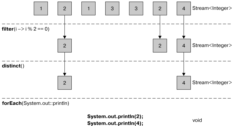
Рис. 5.2. Фильтрация уникальных элементов потока данных
