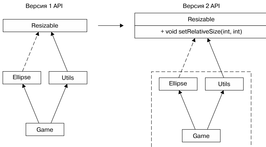
Рис. 13.2. Развитие API путем добавления метода в интерфейс Resizable . Повторная компиляция приложения приводит к ошибкам, поскольку оно зависит от интерфейса Resizable
