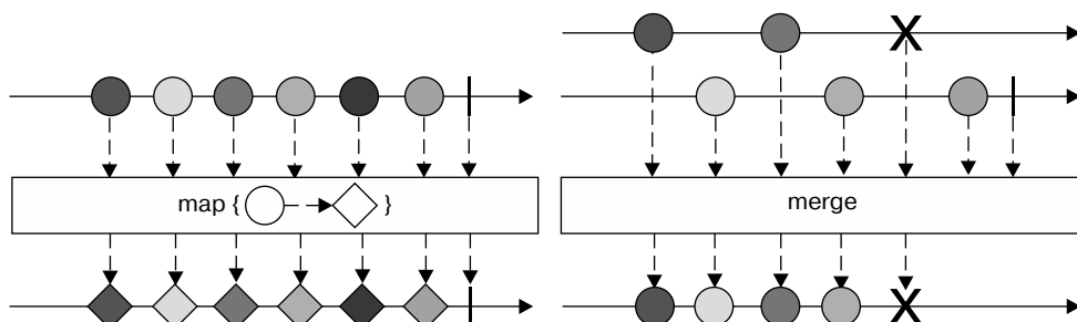
Рис. 17.5. «Мраморные» диаграммы для функций map и merge
