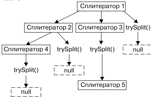
Рис. 7.6. Рекурсивный процесс разбиения
