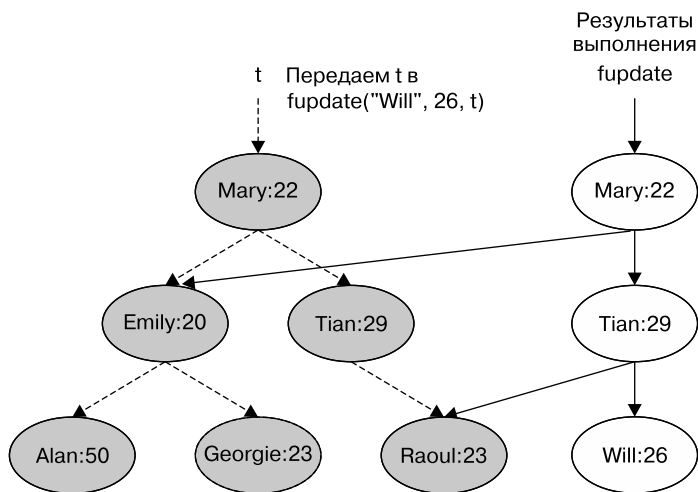
Рис. 19.4. При выполнении этого обновления дерева ни одна существующая структура данных не пострадала
