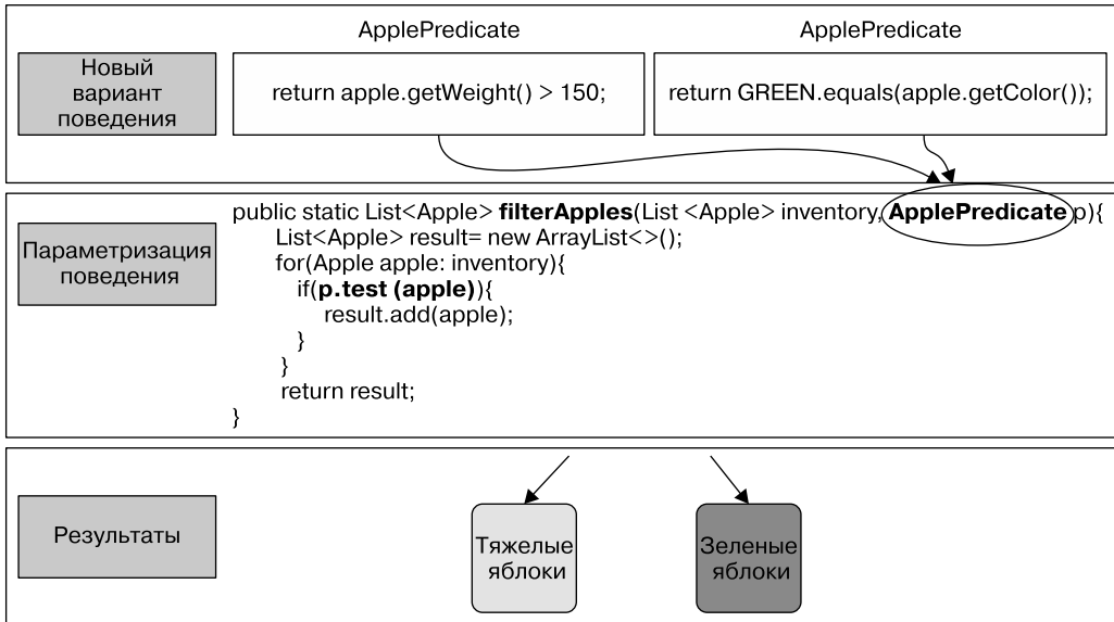
Рис. 2.3. Параметризация поведения метода filterApples и передача ему различных стратегий фильтрации
