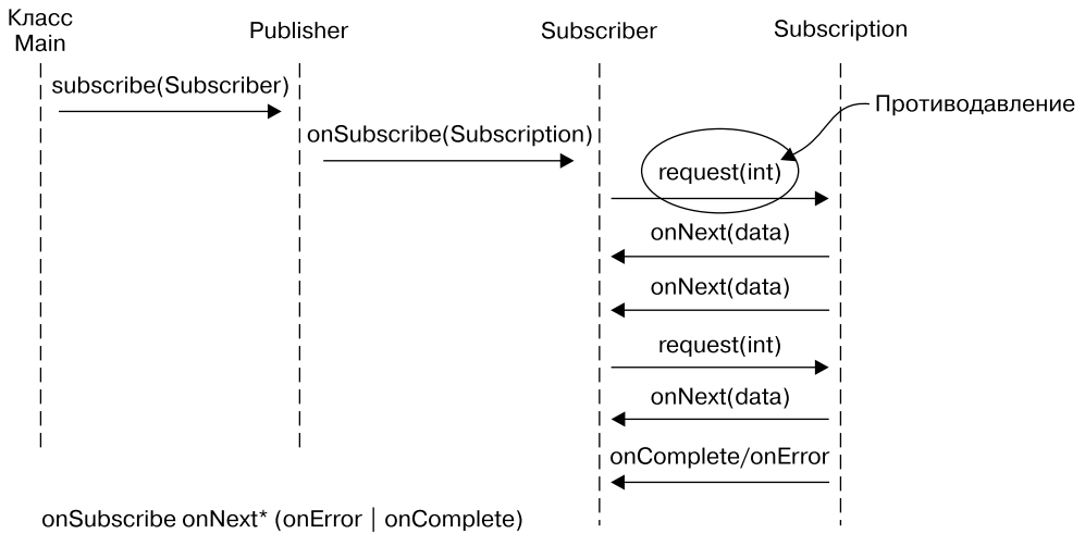
Рис. 17.3. Жизненный цикл реактивного приложения, использующего Flow API
