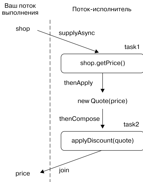
Рис. 16.3. Композиция синхронных и асинхронных операций
