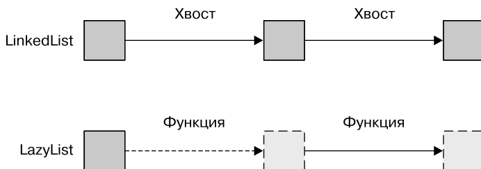
Рис. 19.5. Элементы LinkedList уже существуют в оперативной памяти (разнесены по ней). А элементы LazyList создаются функцией по требованию; их можно рассматривать как разнесенные во времени
