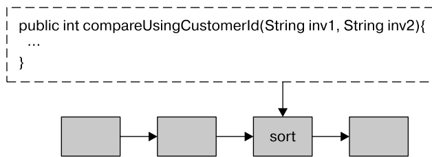
Рис. 1.3. Передача метода compareUsingCustomerId в виде аргумента методу sort
