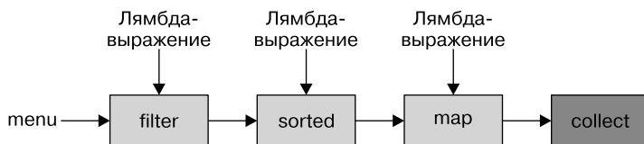
Рис. 4.1. Создание конвейера потоковой обработки с помощью соединения потоковых операций цепочкой
