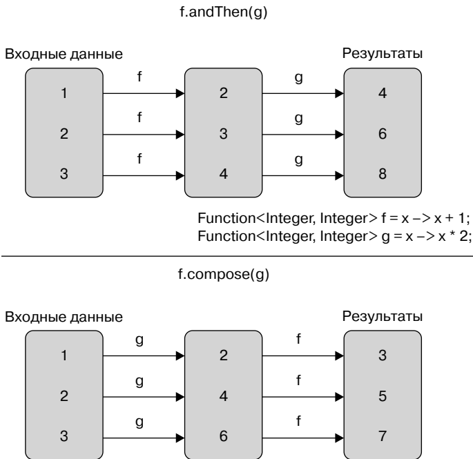
Рис. 3.6. andThen по сравнению с compose
