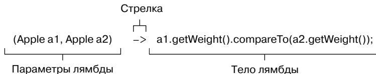
Рис. 3.1. Лямбда-выражение состоит из параметров, стрелки и тела
