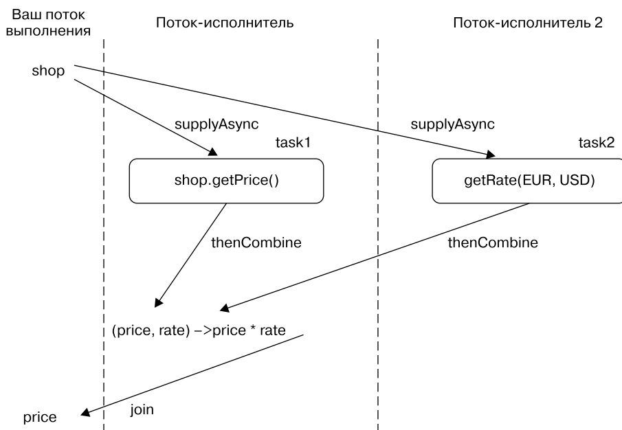
Рис. 16.4. Сочетание двух независимых асинхронных задач
