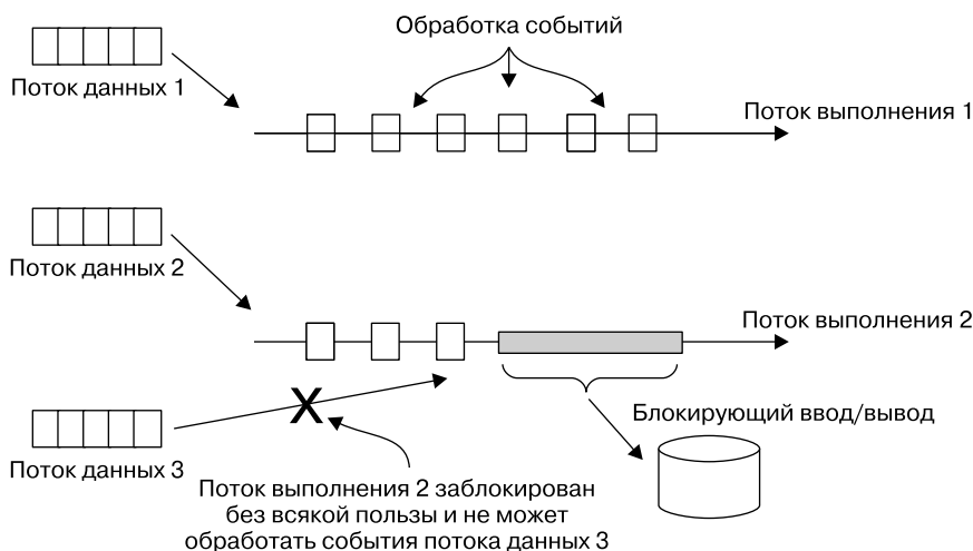
Рис. 17.2. Блокирующая операция удерживает без всякой пользы поток выполнения, в результате чего он не может производить другие вычисления
