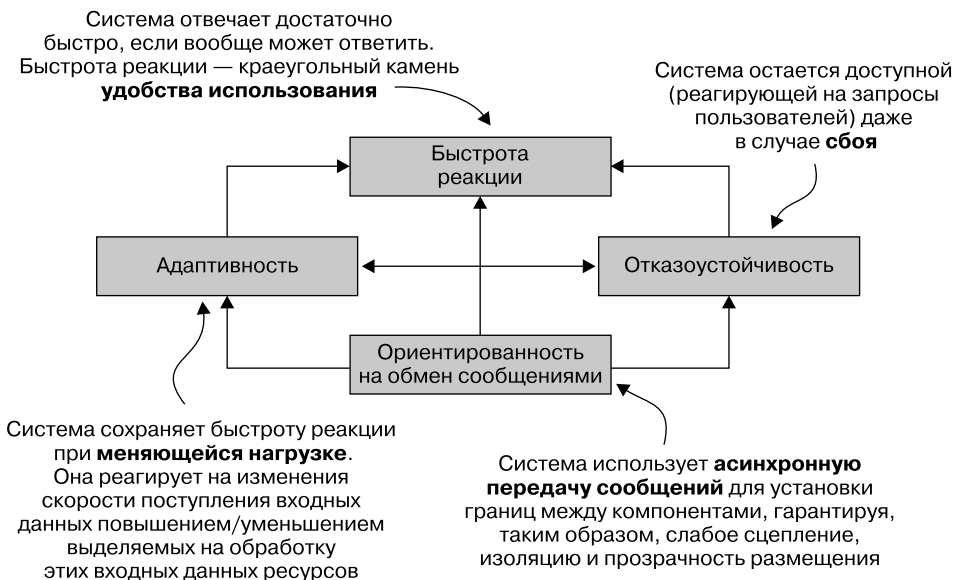
Рис. 17.1. Ключевые особенности реактивных систем
