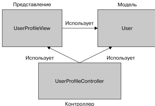
Рис. 14.1. Три отдельные зоны ответственности и зависимости между ними
