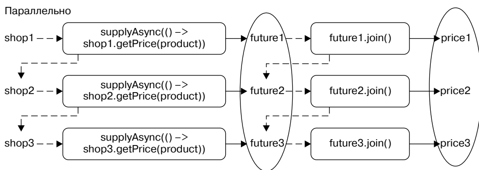
Рис. 16.2. Почему отложенная природа потоков данных приводит к последовательному выполнению вычислений и как этого избежать
