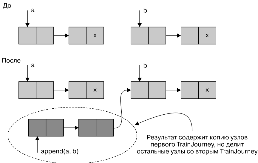
Рис. 19.3. Функциональный стиль без модификаций структуры данных
