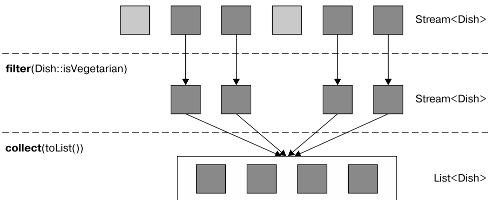
Рис. 5.1. Фильтрация потока данных с помощью предиката
