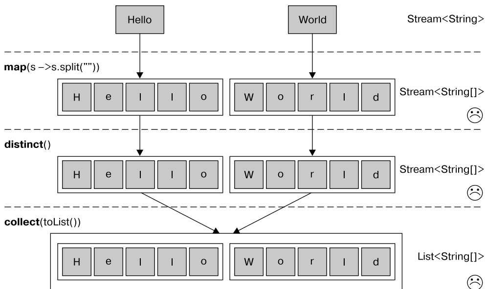
Рис. 5.5. Неправильное использование метода map для получения уникальных символов из списка слов
