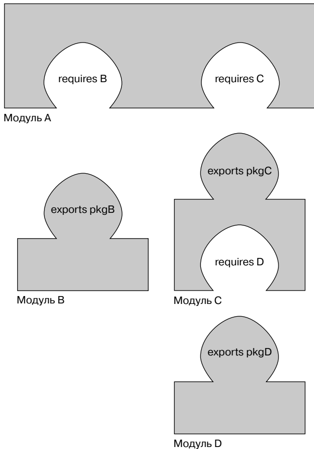
Рис. 14.3. Пример Java-системы из четырех модулей (А, В, С, D) в стиле пазла. Для модуля А нужны модули В и С, поэтому ему требуется доступ к пакетам pkgB и pkgC (экспортируемым модулями В и С соответственно). Аналогично модуль С может использовать пакет pkgD, а модуль В — нет
