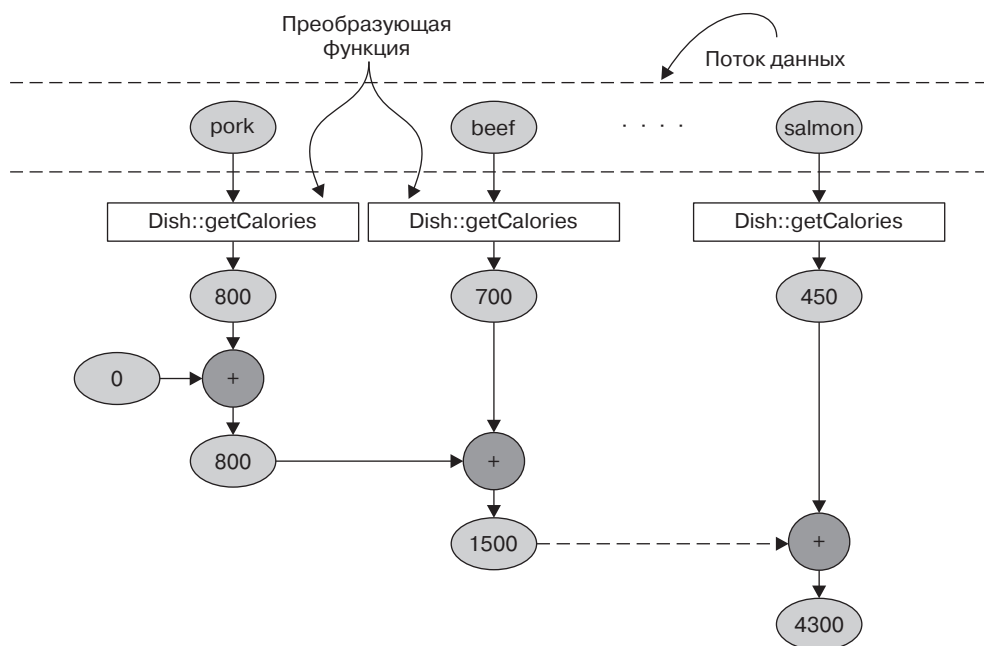
Рис. 6.2. Процесс агрегирования при использовании коллектора summingInt
