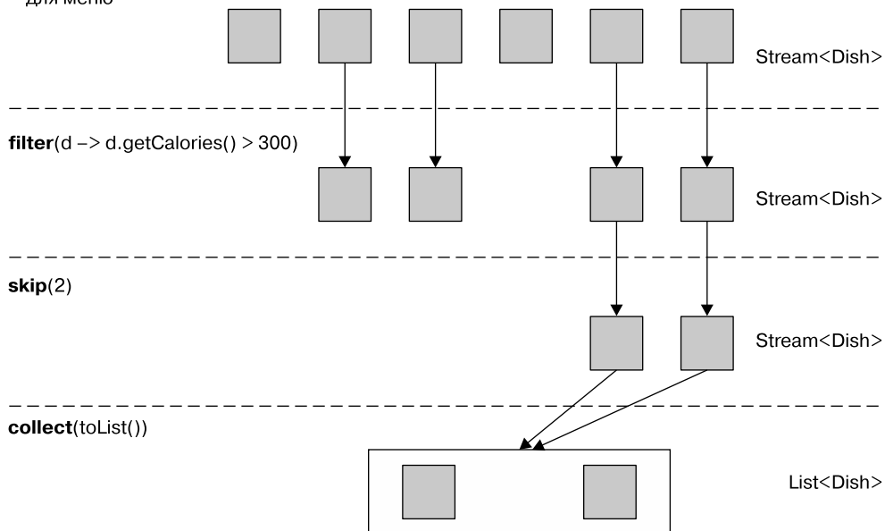
Рис. 5.4. Пропуск элементов потока данных
