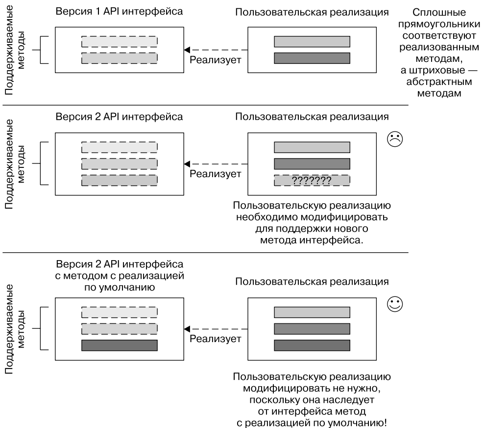
Рис. 13.1. Добавление метода в интерфейс
