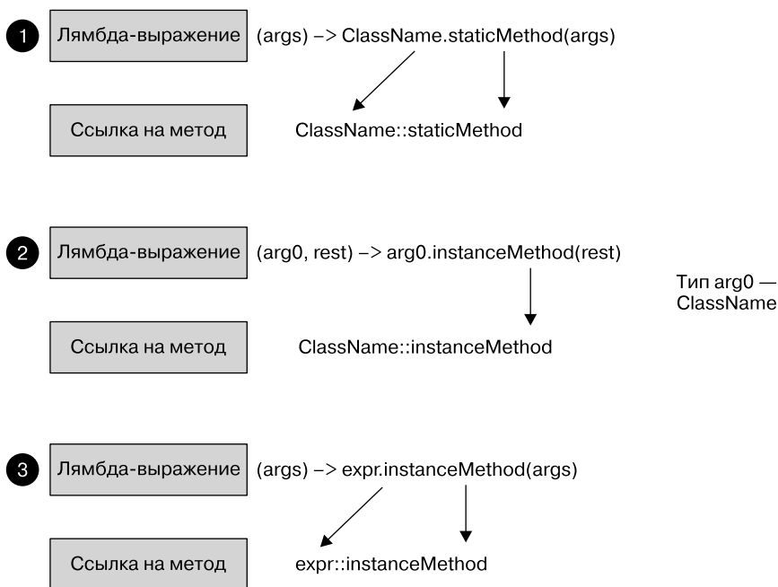
Рис. 3.5. Инструкции по конструированию ссылок на методы для трех различных типов лямбда-выражений
