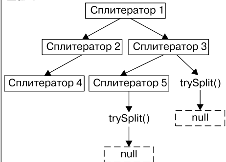
Рис. 7.6. Рекурсивный процесс разбиения
