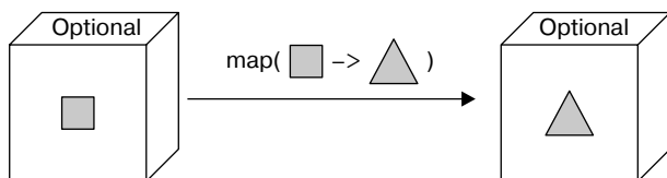
Рис. 11.2. Сравнение методов map интерфейса Stream и класса Optional
