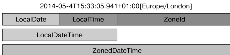
Рис. 12.1. Разбираемся с ZonedDateTime
