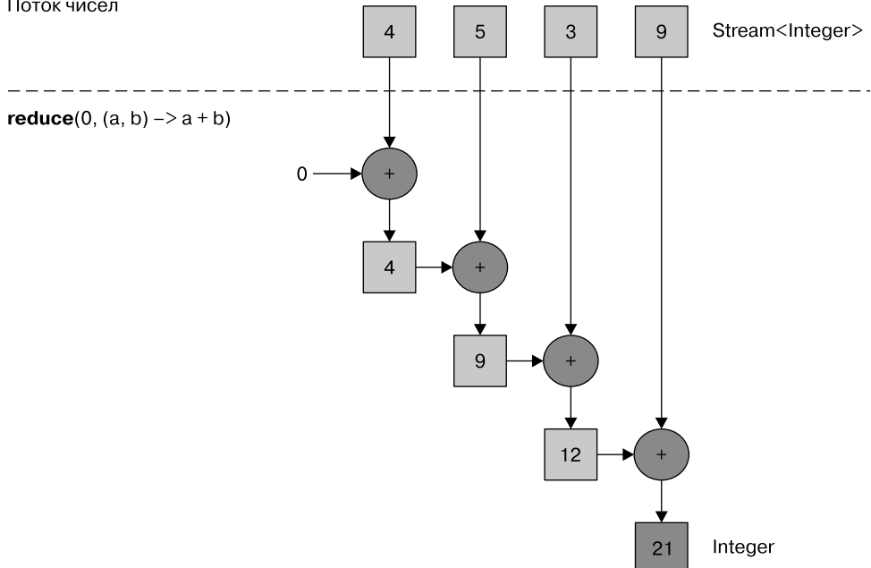
Рис. 5.7. Использование метода reduce для суммирования чисел из потока данных
