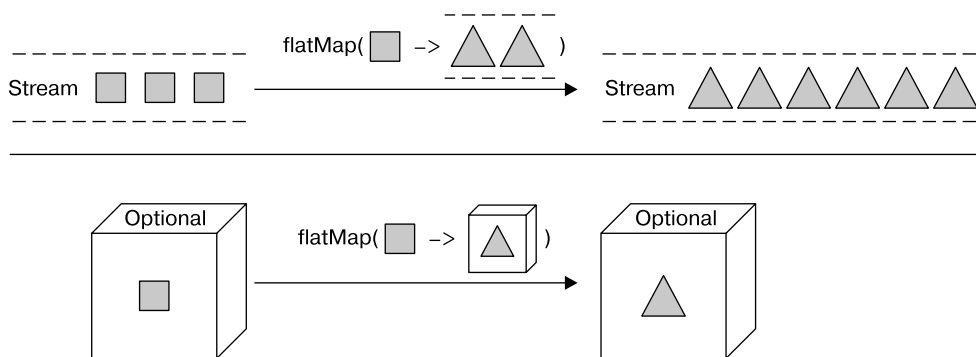
Рис. 11.4. Сравнение методов flatMap интерфейса Stream и класса Optional
