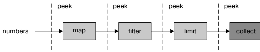
Рис. 9.4. Просмотр проходящих через поток данных значений с помощью операции peek
