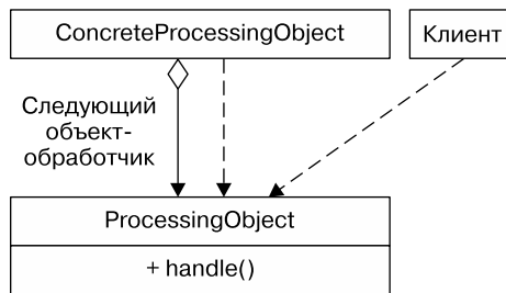
Рис. 9.3. Паттерн проектирования «Цепочка обязанностей»
