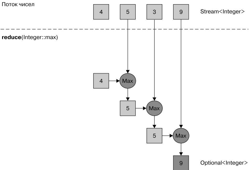
Рис. 5.8. Операция reduce — вычисление максимума
