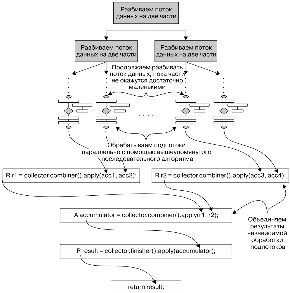
Рис. 6.8. Распараллеливание процесса свертки с помощью метода combiner
