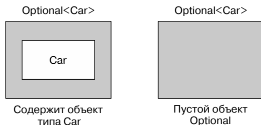
Рис. 11.1. Опционал Car
