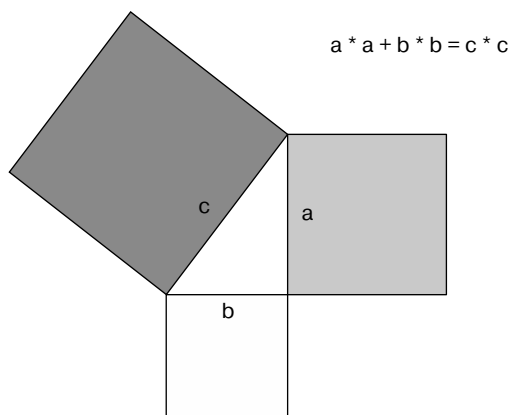
Рис. 5.9. Теорема Пифагора
