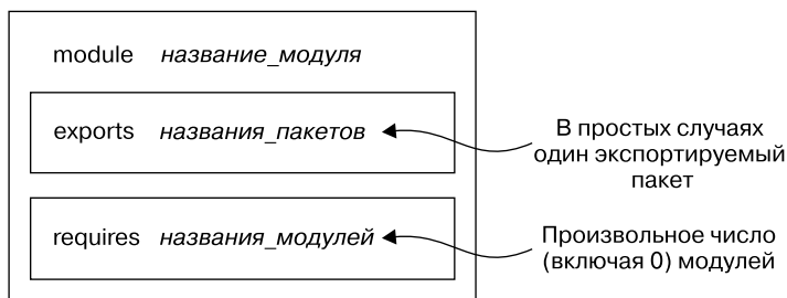
Рис. 14.2. Базовая структура дескриптора модуля Java ( module-info.java )
