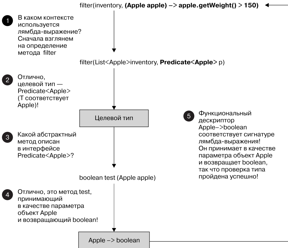
Рис. 3.4. Пошаговый разбор процесса проверки типа лямбда-выражения
