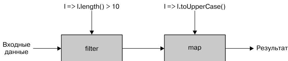
Рис. 20.1. Потокотипные операции над списками в языке Scala
