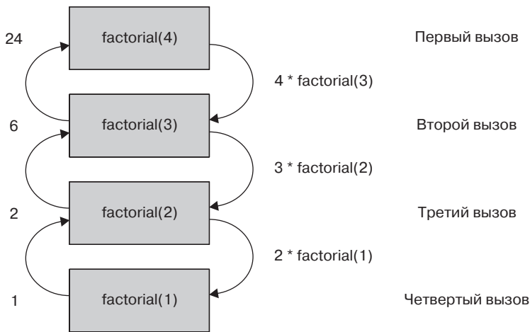
Рис. 18.5. Рекурсивное определение факториала, требующее нескольких фреймов стека
