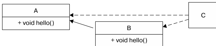
Рис. 13.5. Преимущество — у самого конкретного из содержащих реализацию по умолчанию интерфейсов
