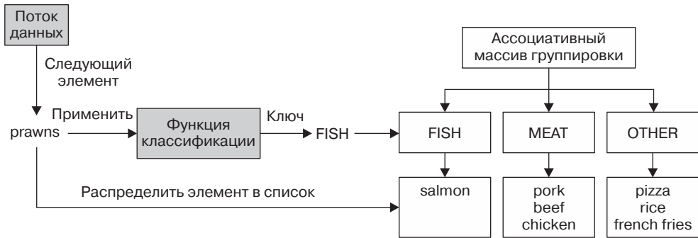
Рис. 6.4. Классификация элементов потока в процессе группировки
