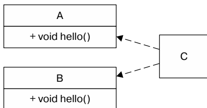
Рис. 13.7. Реализует два интерфейса
