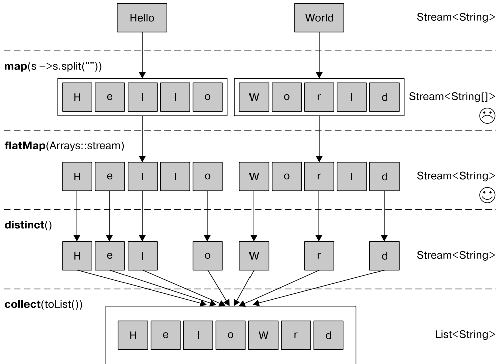
Рис. 5.6. Использование метода flatMap для получения уникальных символов из списка слов
