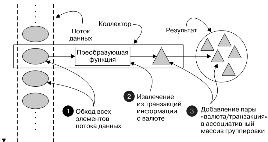
Рис. 6.1. Процесс свертки: группировка транзакций по валюте
