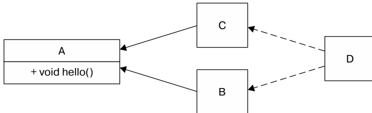
Рис. 13.8. Проблема ромбовидного наследования
