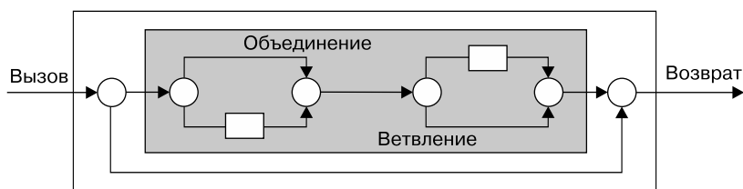
Рис. 15.4. Строгое ветвление-объединение. Стрелки соответствуют потокам выполнения, окружности — ветвлениям и объединениям, а прямоугольники отражают вызовы методов и возвраты из них
