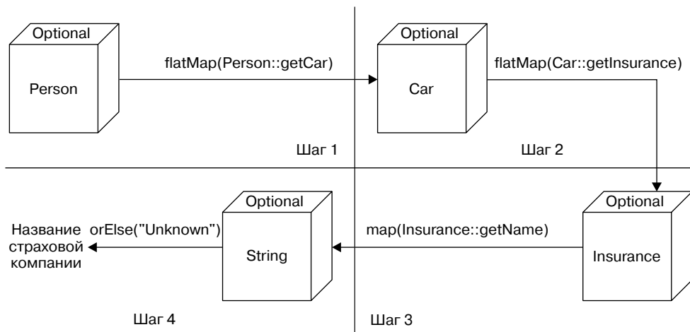
Рис. 11.5. Цепочка разыменования Person/Car/Insurance с использованием опционалов
