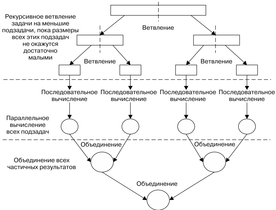
Рис. 7.3. Процесс ветвления-объединения
