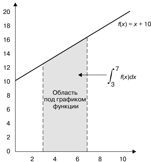
Рис. 3.8. Область под графиком функции f(x) = x + 10 для x от 3 до 7
