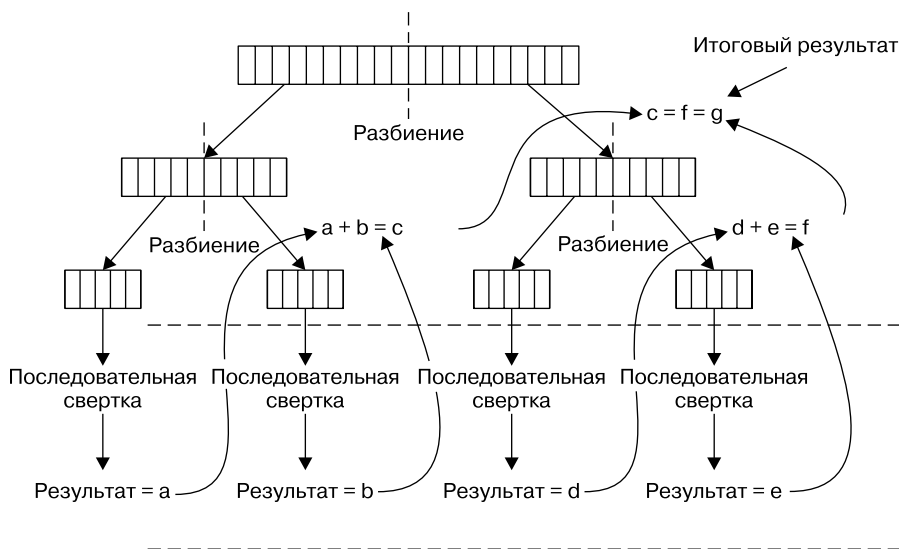
Рис. 7.4. Алгоритм ветвления-объединения
