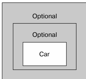
Рис. 11.3. Двухуровневый опционал
