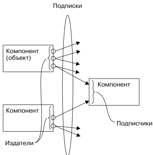
Рис. 15.9. Модель публикации/подписки
