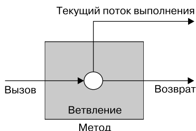
Рис. 15.6. Асинхронный метод
