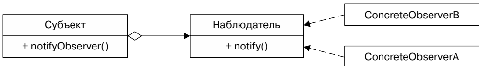
Рис. 9.2. Паттерн проектирования «Наблюдатель»
