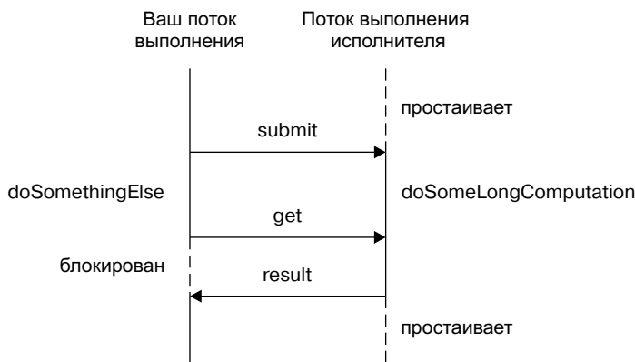
Рис. 16.1. Применение фьючерсов для асинхронного выполнения «долгоиграющих» операций
