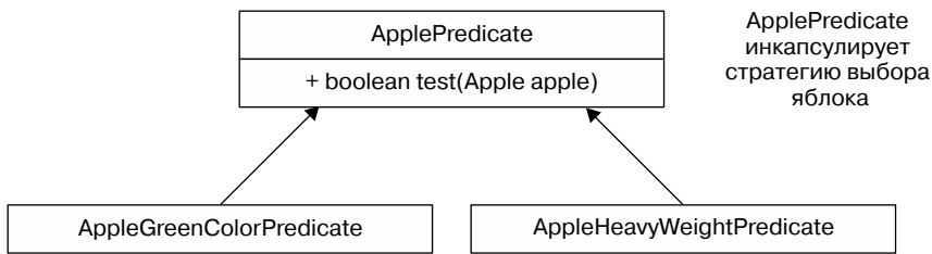
Рис. 2.1. Различные стратегии выбора объектов Apple
