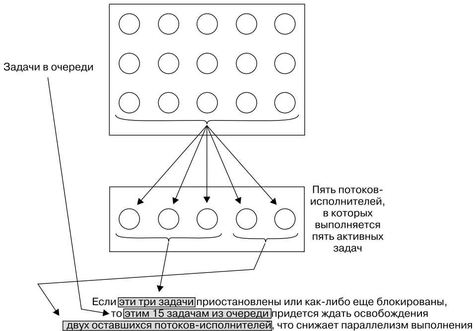
Рис. 15.3. Приостановленные задачи снижают пропускную способность пулов потоков выполнения
